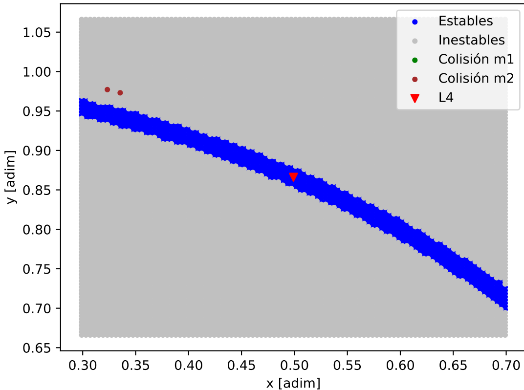
Mapa de estabilidad - HD_148164_HD_148164_b
