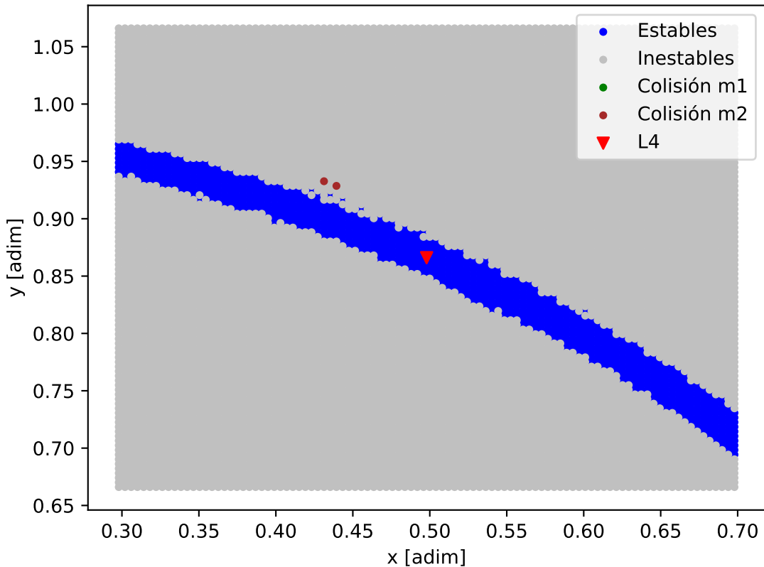
Mapa de estabilidad - HD_169830_HD_169830_b
