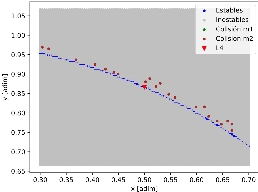
Mapa de estabilidad - HD_217786_HD_217786_c
