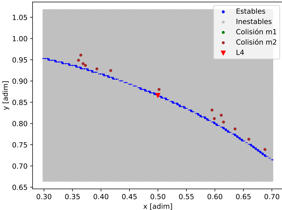
Mapa de estabilidad - HD_22946_TOI-411_b
