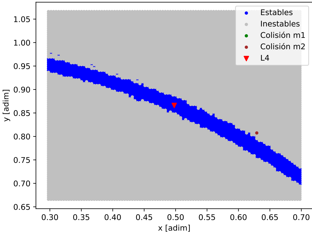
Mapa de estabilidad - HD_23079_HD_23079_b
