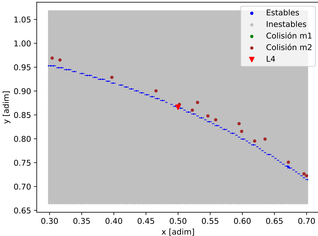
Mapa de estabilidad - HD_28109_HD_28109_b
