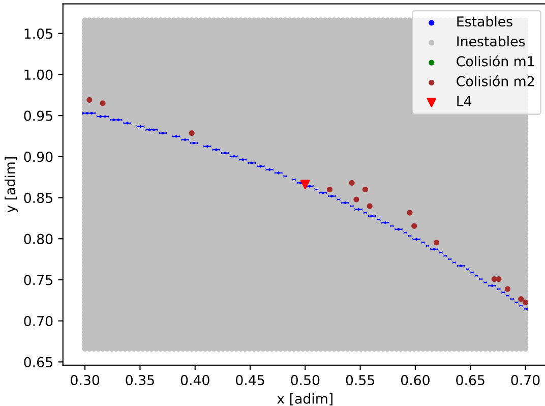
Mapa de estabilidad - HD_28109_HD_28109_d
