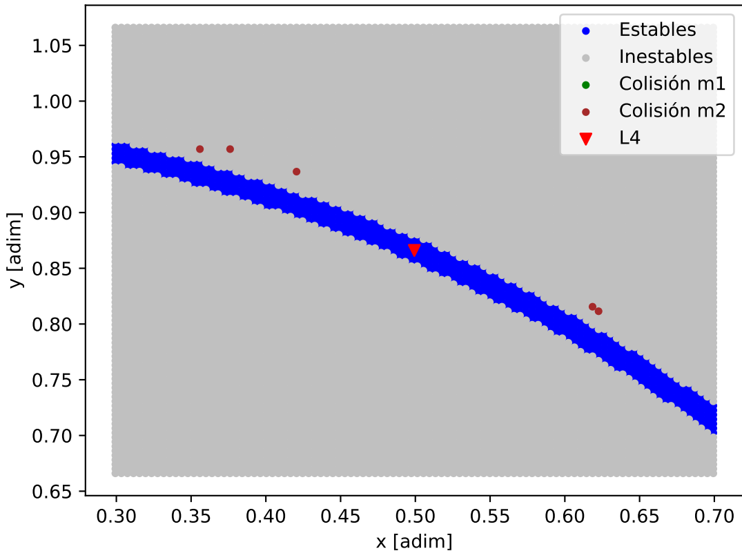
Mapa de estabilidad - HD_60532_HD_60532_b
