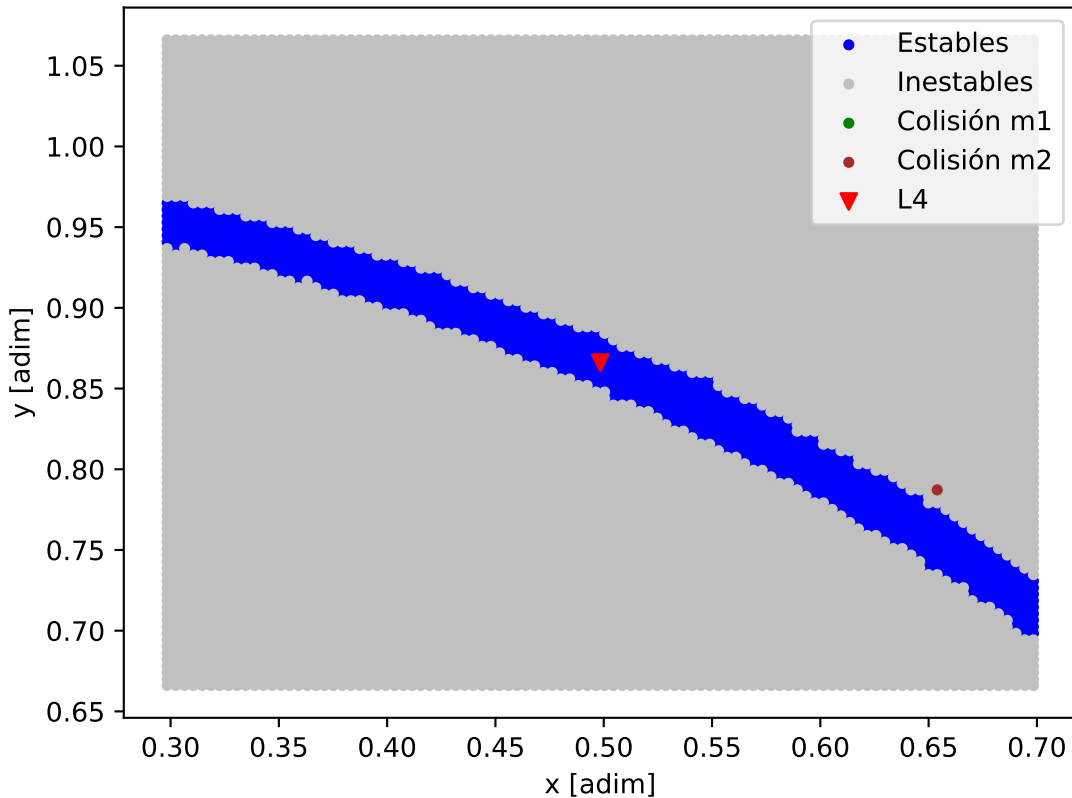
Mapa de estabilidad - HD_60532_HD_60532_c
