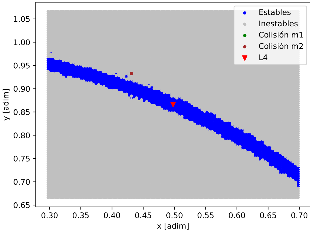
Mapa de estabilidad - HD_67087_HD_67087_b
