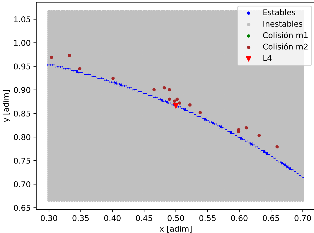
Mapa de estabilidad - HD_73344_HD_73344_b
