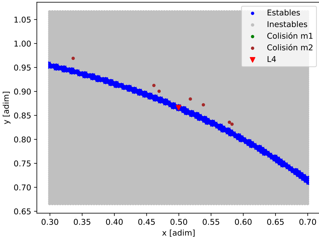
Mapa de estabilidad - HD_73344_HD_73344_c
