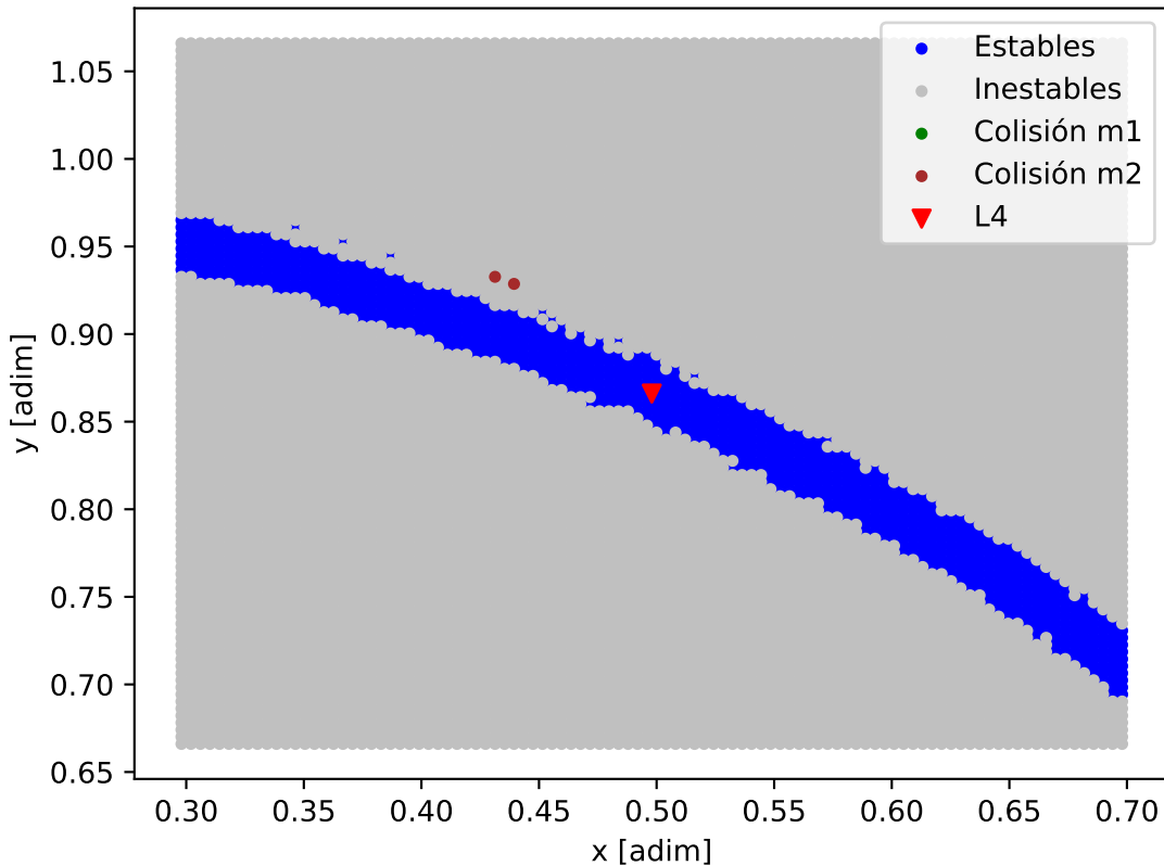
Mapa de estabilidad - HD_73344_HD_73344_d
