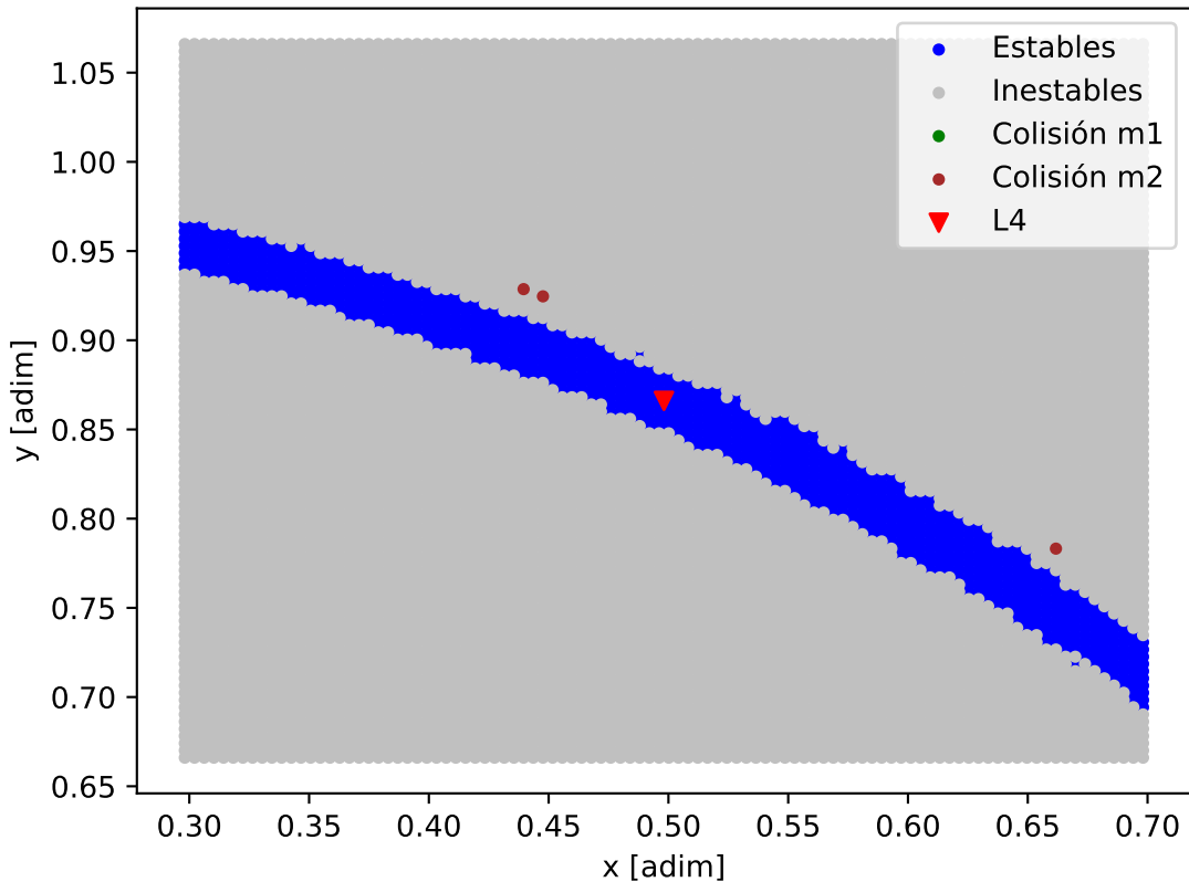
Mapa de estabilidad - HD_75898_HD_75898_b
