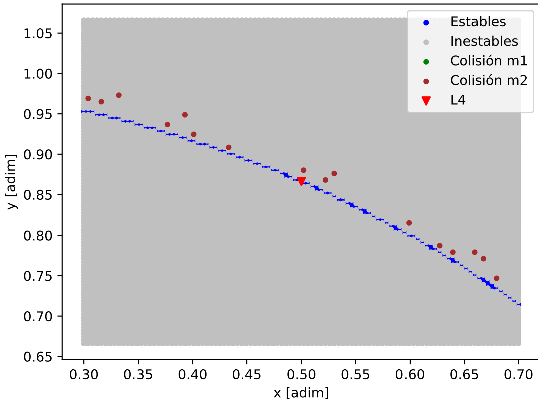
Mapa de estabilidad - HIP_41378_HIP_41378_b
