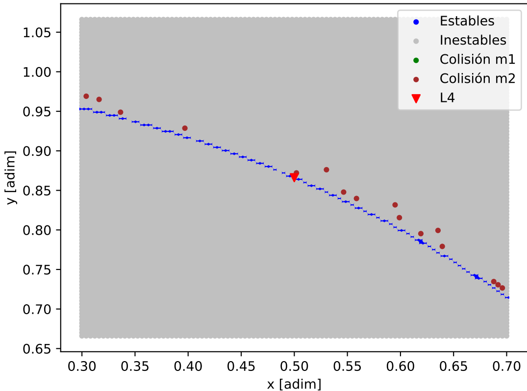
Mapa de estabilidad - HIP_41378_HIP_41378_c
