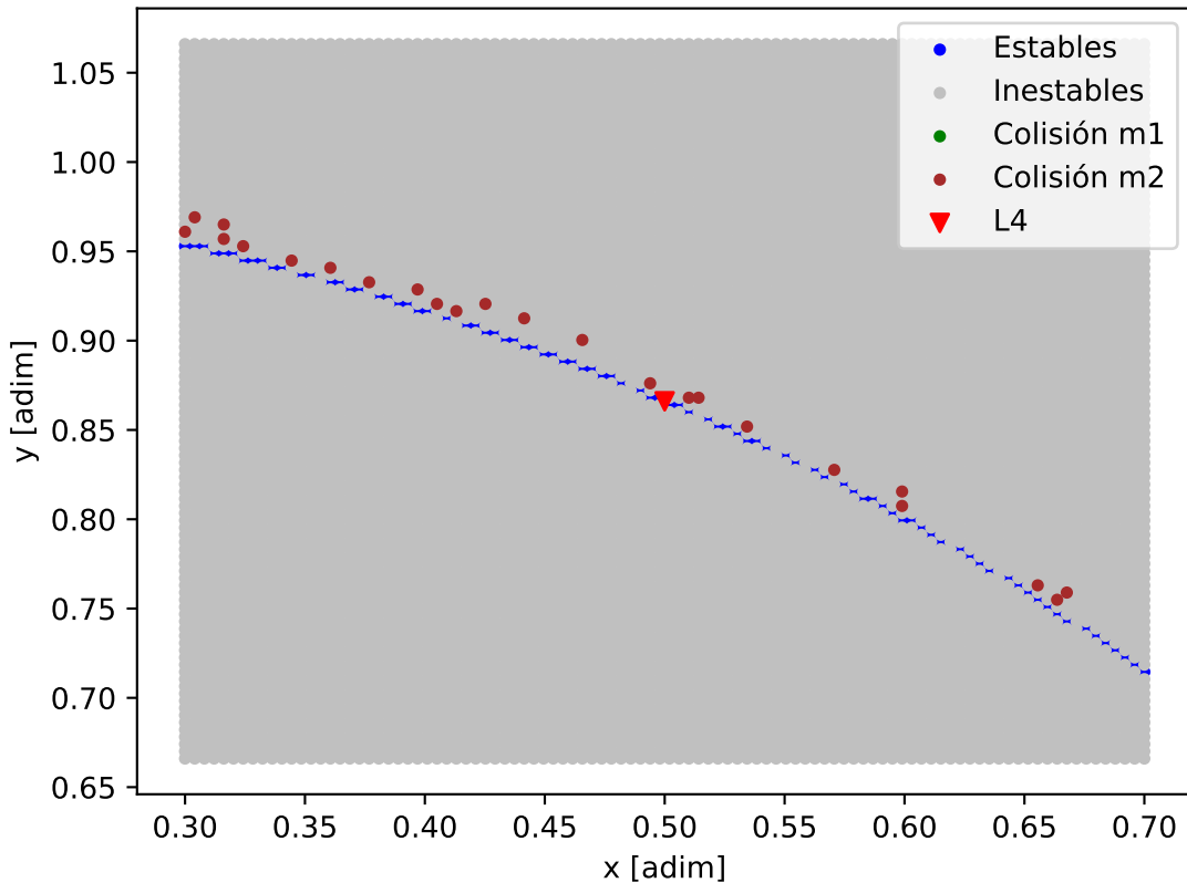
Mapa de estabilidad - HR_858_HR_858_b
