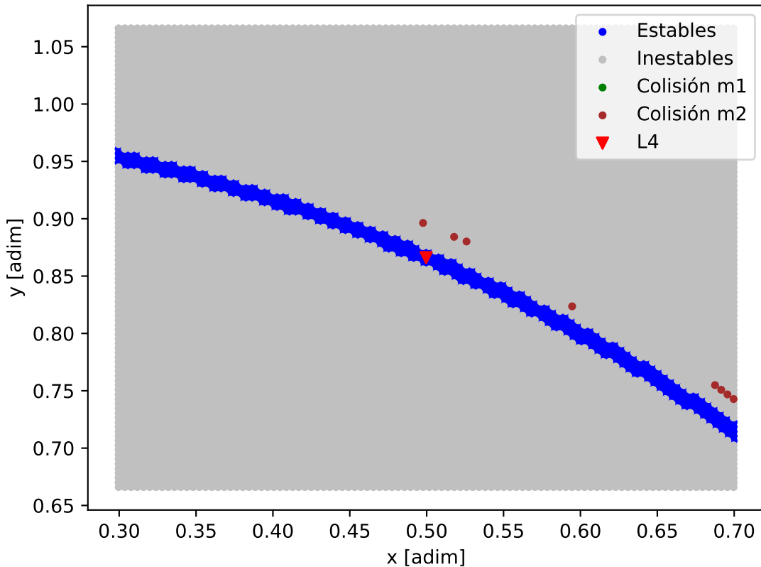
Mapa de estabilidad - KELT-6_KELT-6_b
