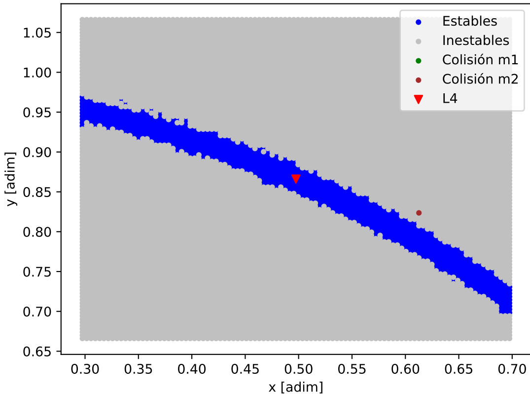
Mapa de estabilidad - KELT-6_KELT-6_c
