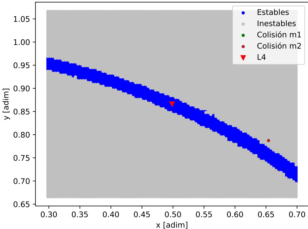
Mapa de estabilidad - Kepler-117_Kepler-117_c
