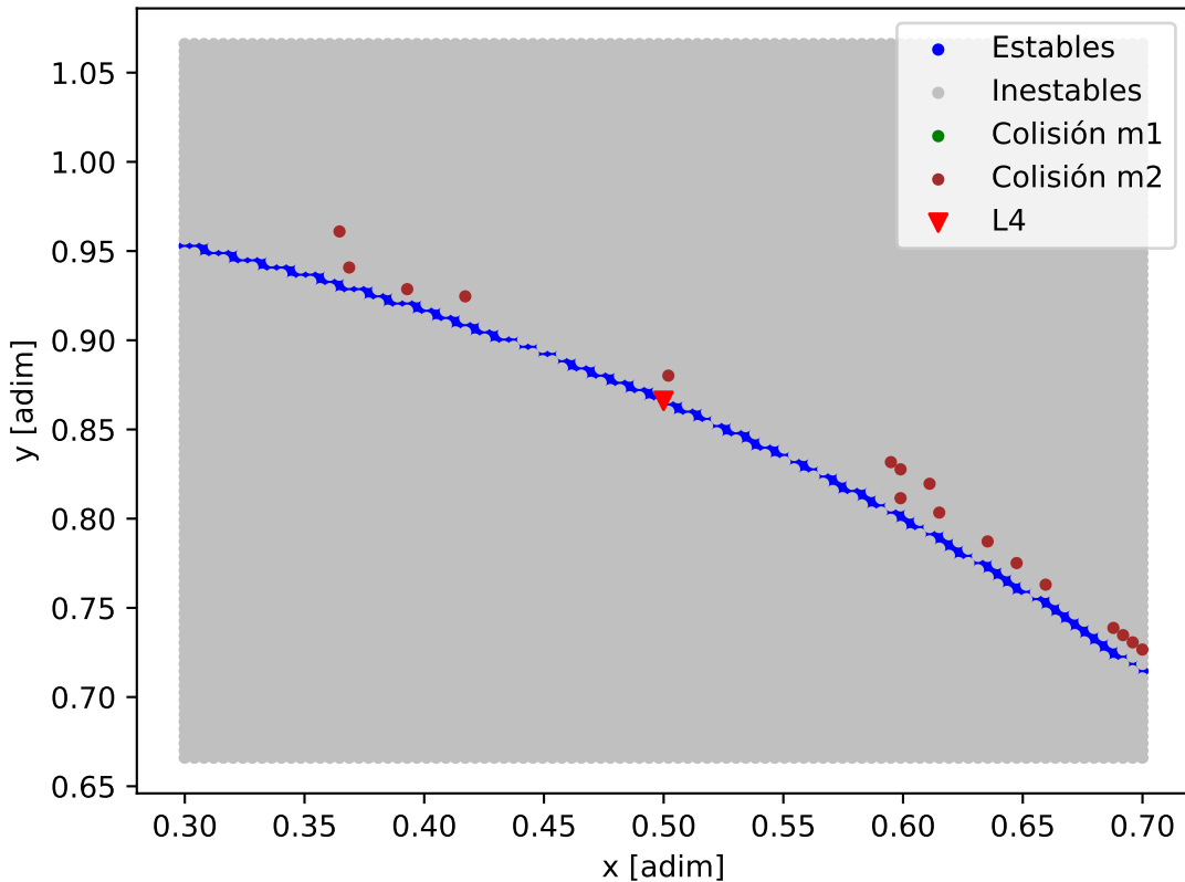
Mapa de estabilidad - Kepler-25_Kepler-25_c
