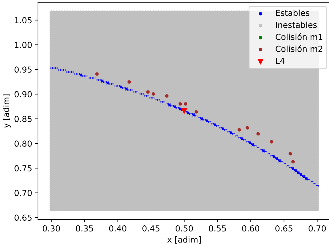
Mapa de estabilidad - TOI-1338_A_TOI-1338_b
