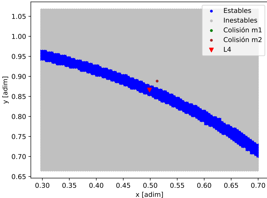
Mapa de estabilidad - TOI-1408_TOI-1408_b
