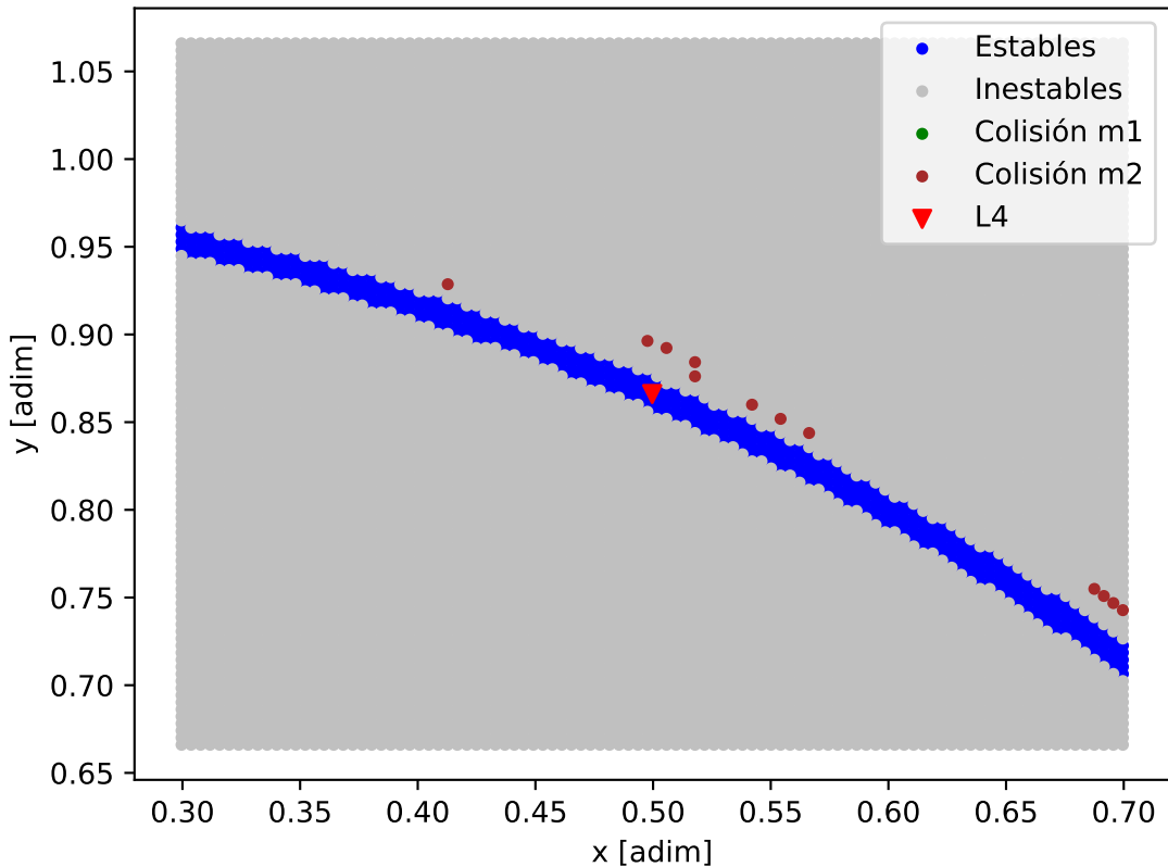
Mapa de estabilidad - TOI-201_TOI-201_b
