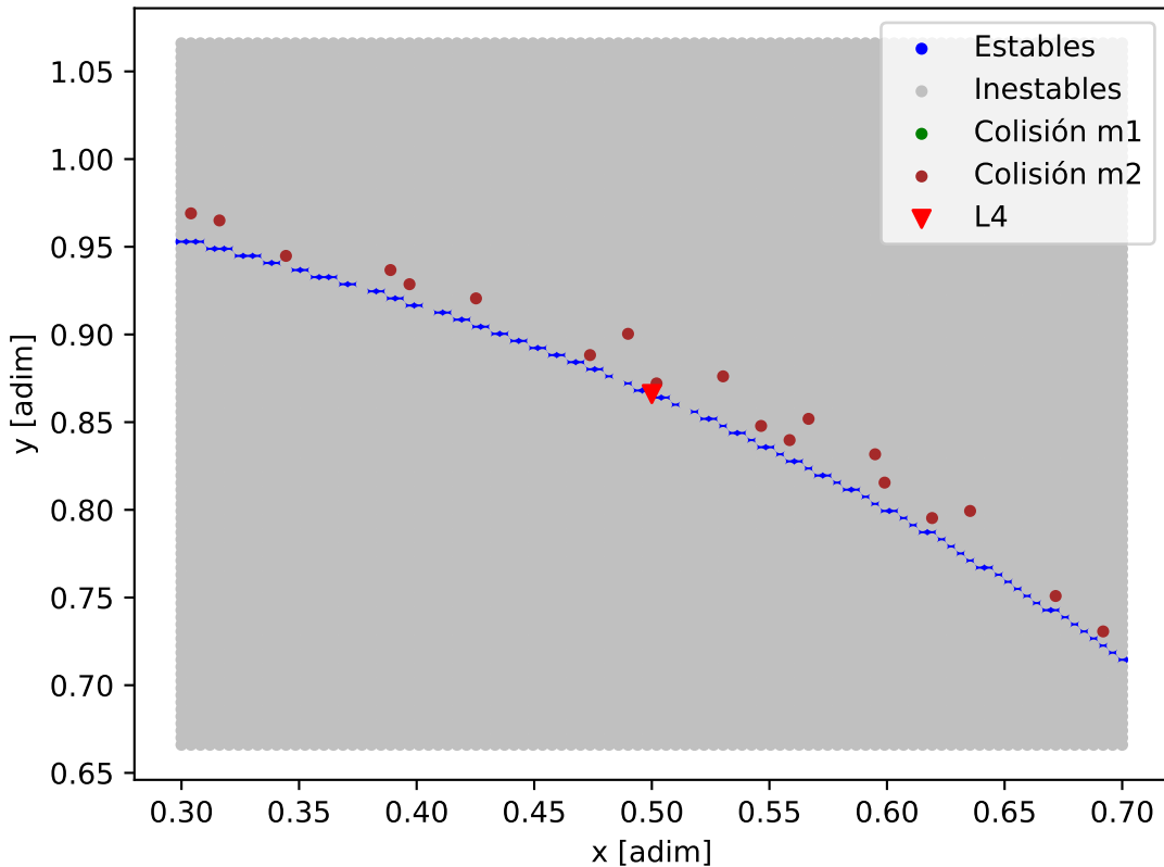
Mapa de estabilidad - TOI-201_TOI-201_d
