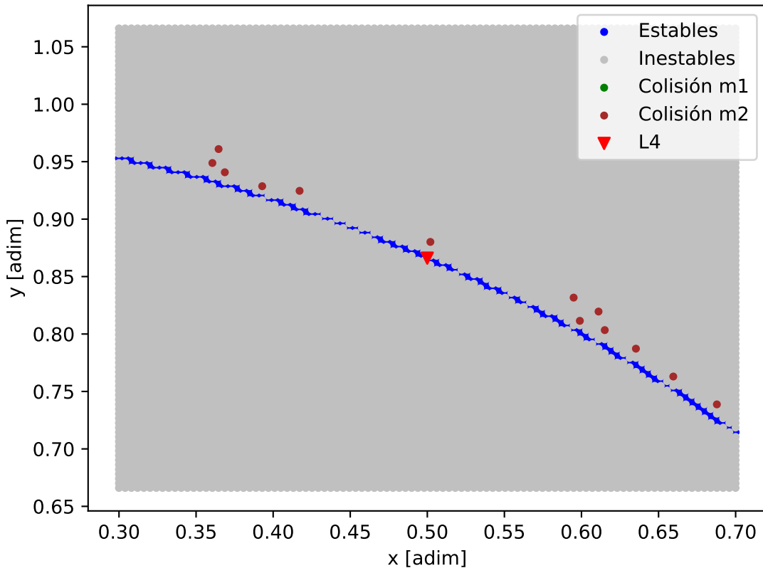
Mapa de estabilidad - TOI-2458_TOI-2458_b
