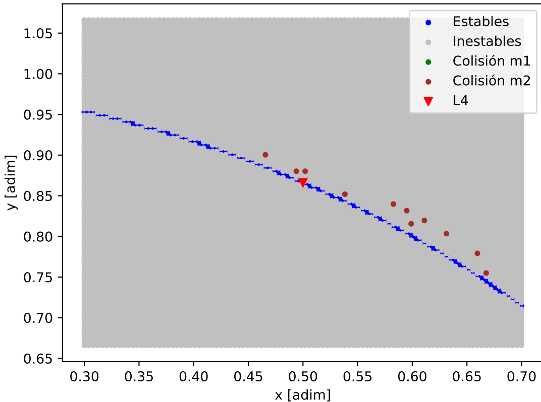
Mapa de estabilidad - TOI-2458_TOI-2458_c
