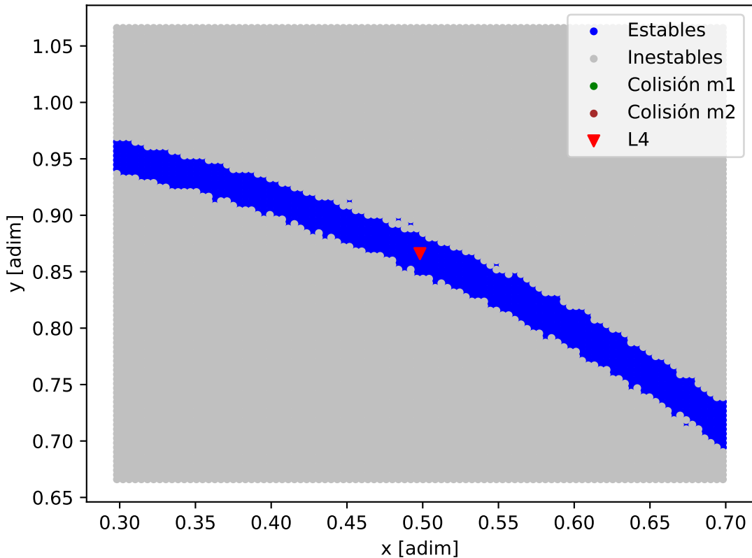
Mapa de estabilidad - TOI-4562_TOI-4562_b
