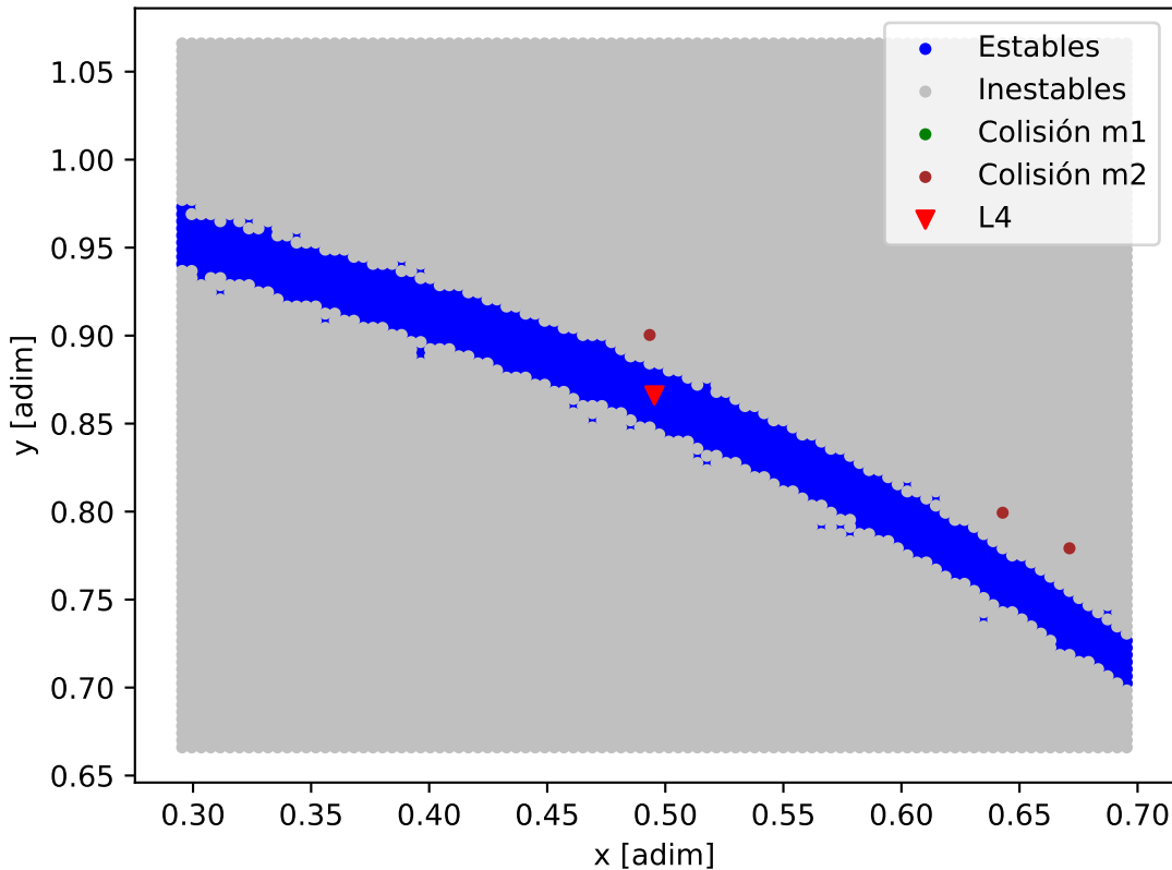
Mapa de estabilidad - TOI-4562_TOI-4562_c
