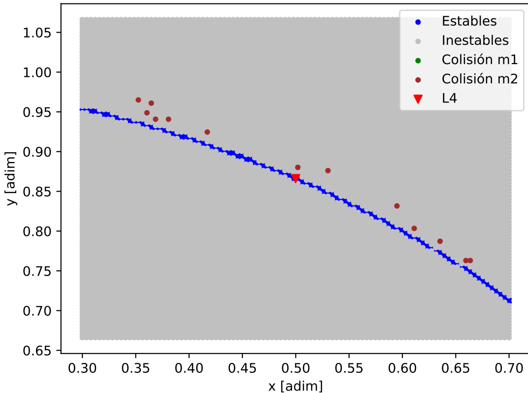
Mapa de estabilidad - TOI-5126_TOI-5126_b
