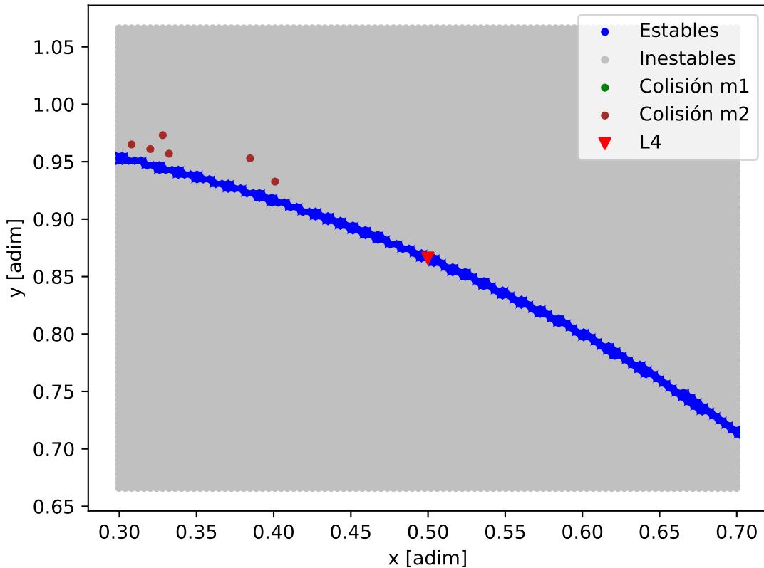
Mapa de estabilidad - TOI-6695_TOI-6695_b
