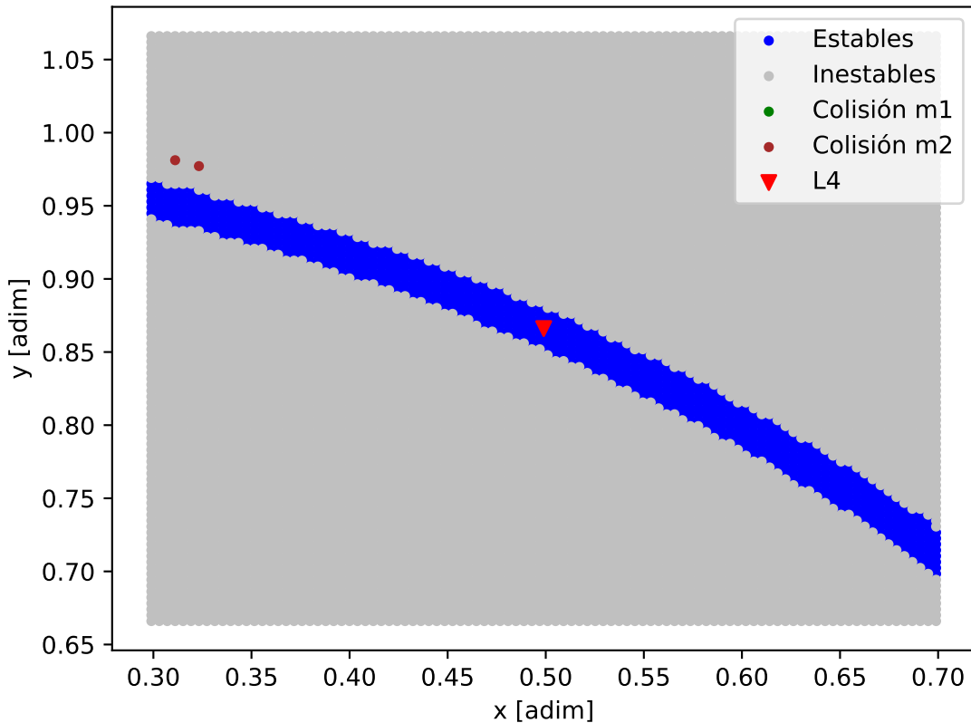
Mapa de estabilidad - TOI-6695_TOI-6695_c
