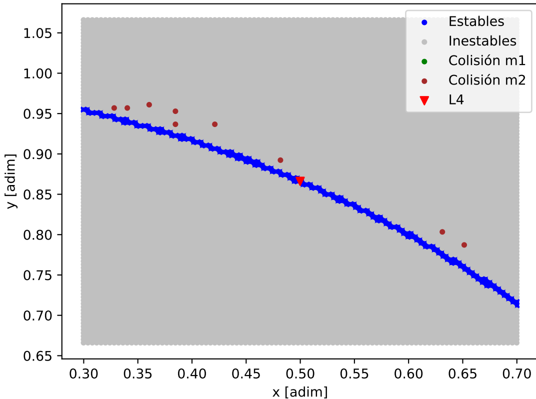
Mapa de estabilidad - WASP-18_WASP-18_c
