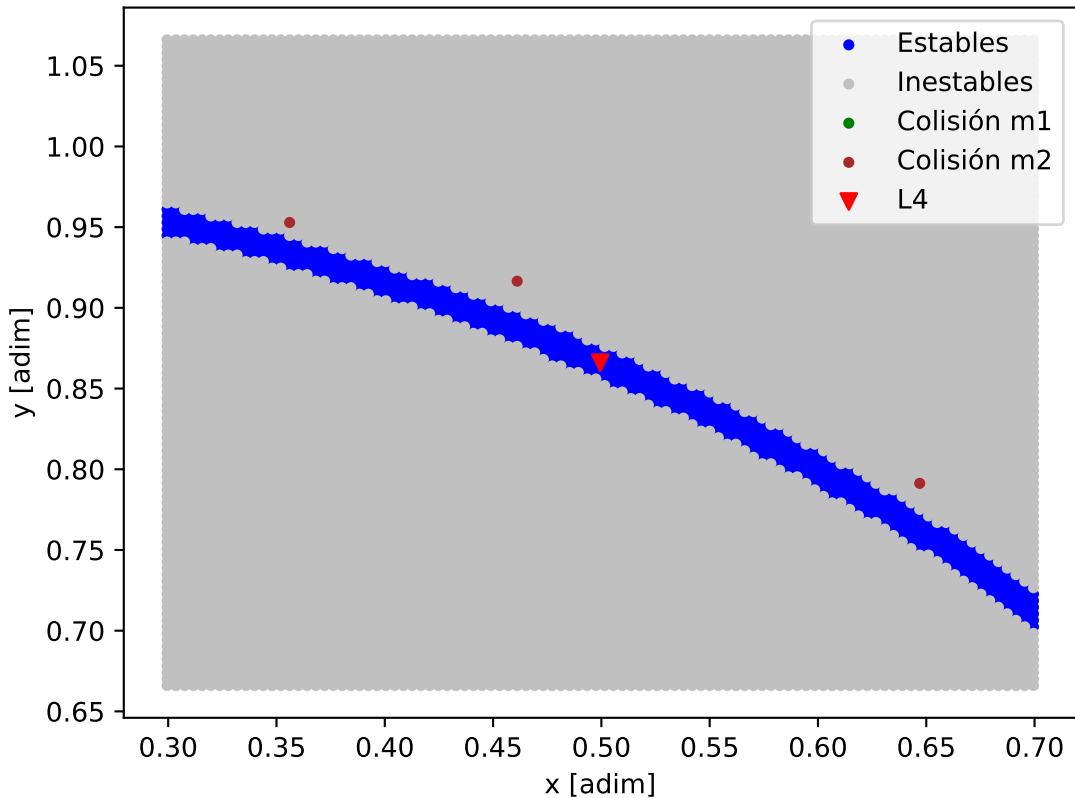
Mapa de estabilidad - ups_And_ups_And_b
