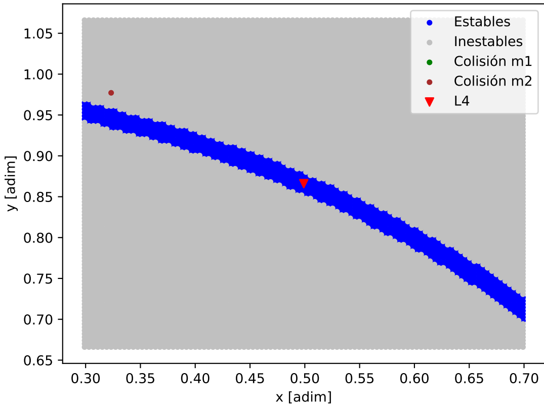
Mapa de estabilidad - BD-11_4672
