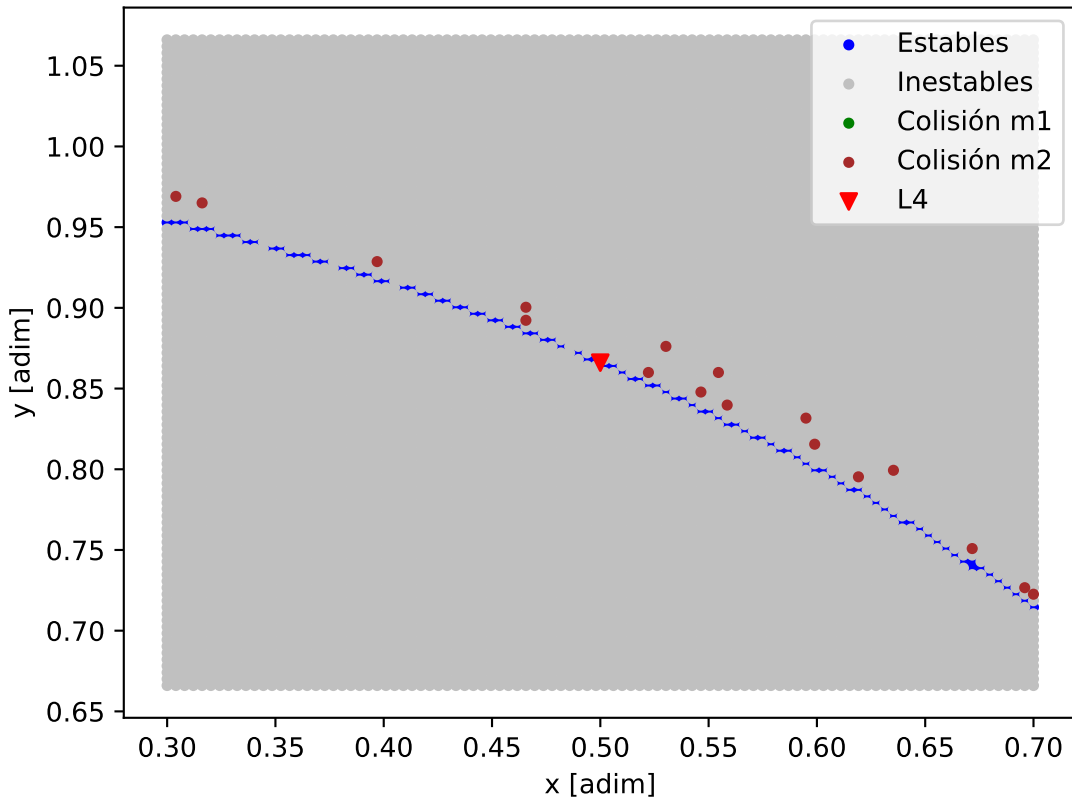
Mapa de estabilidad - GJ_9827
