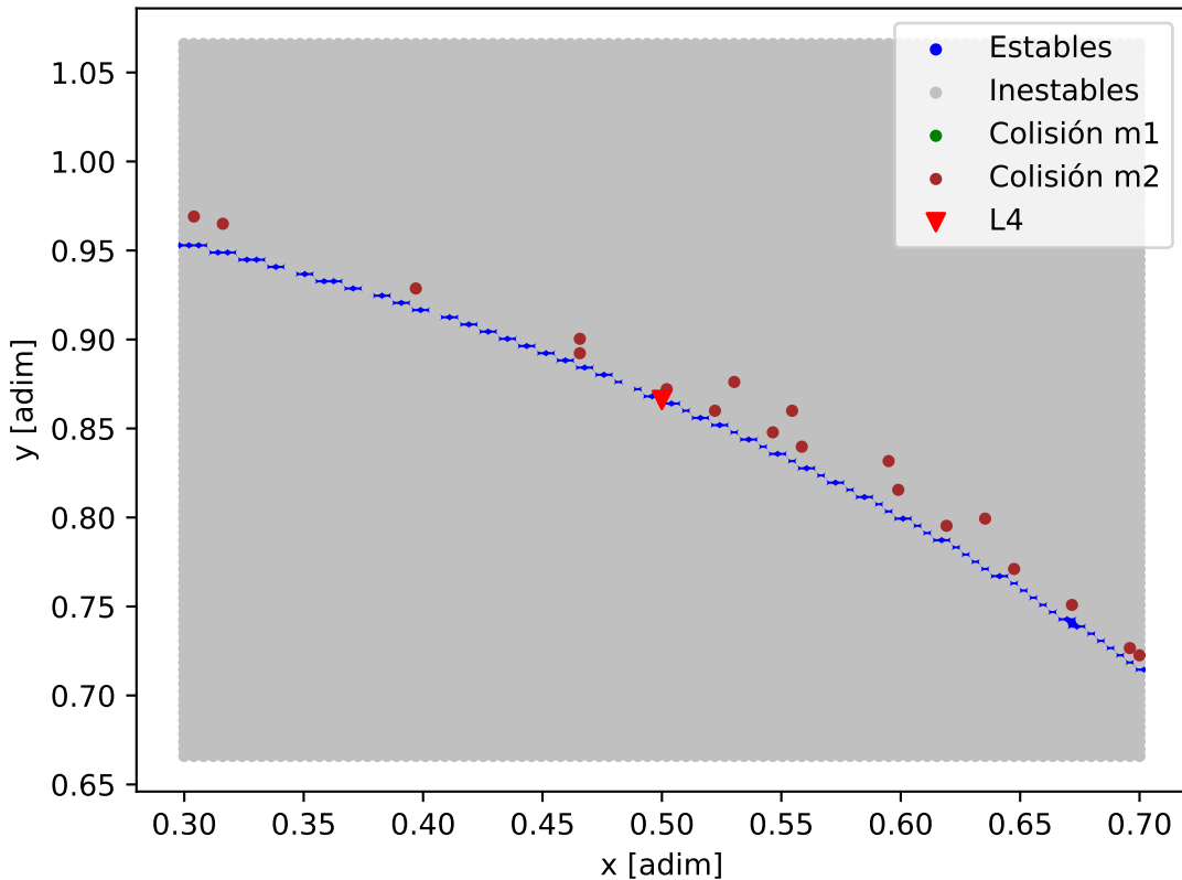
Mapa de estabilidad - HD_110067
