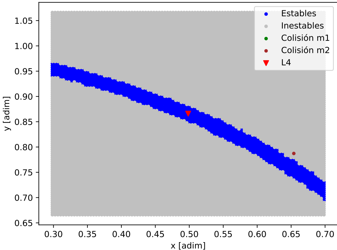
Mapa de estabilidad - HD_118203
