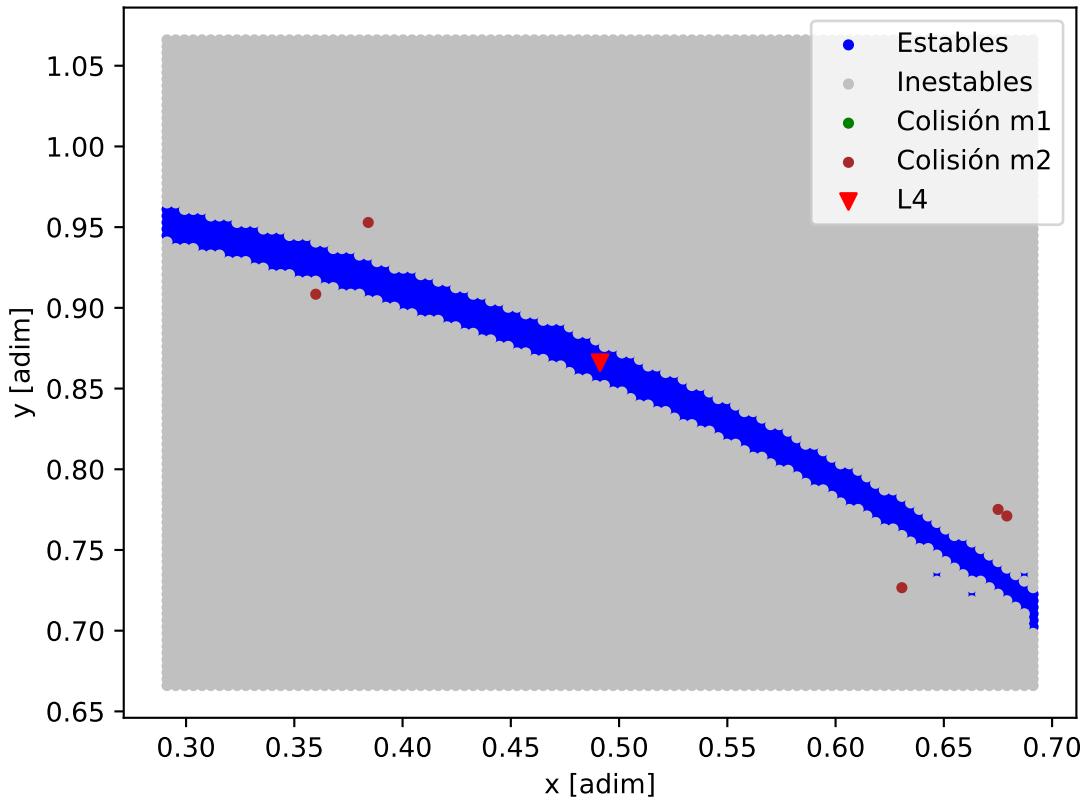
Mapa de estabilidad - HD_118203
