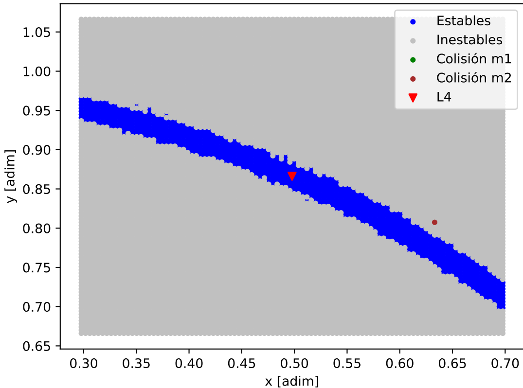
Mapa de estabilidad - HD_12661
