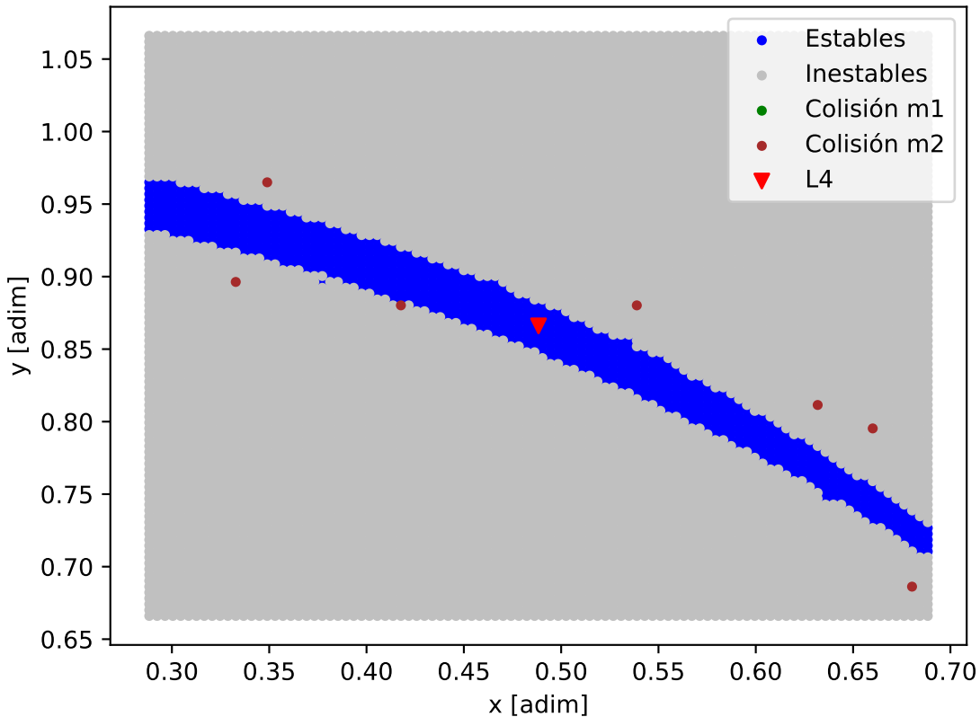
Mapa de estabilidad - HD_164604
