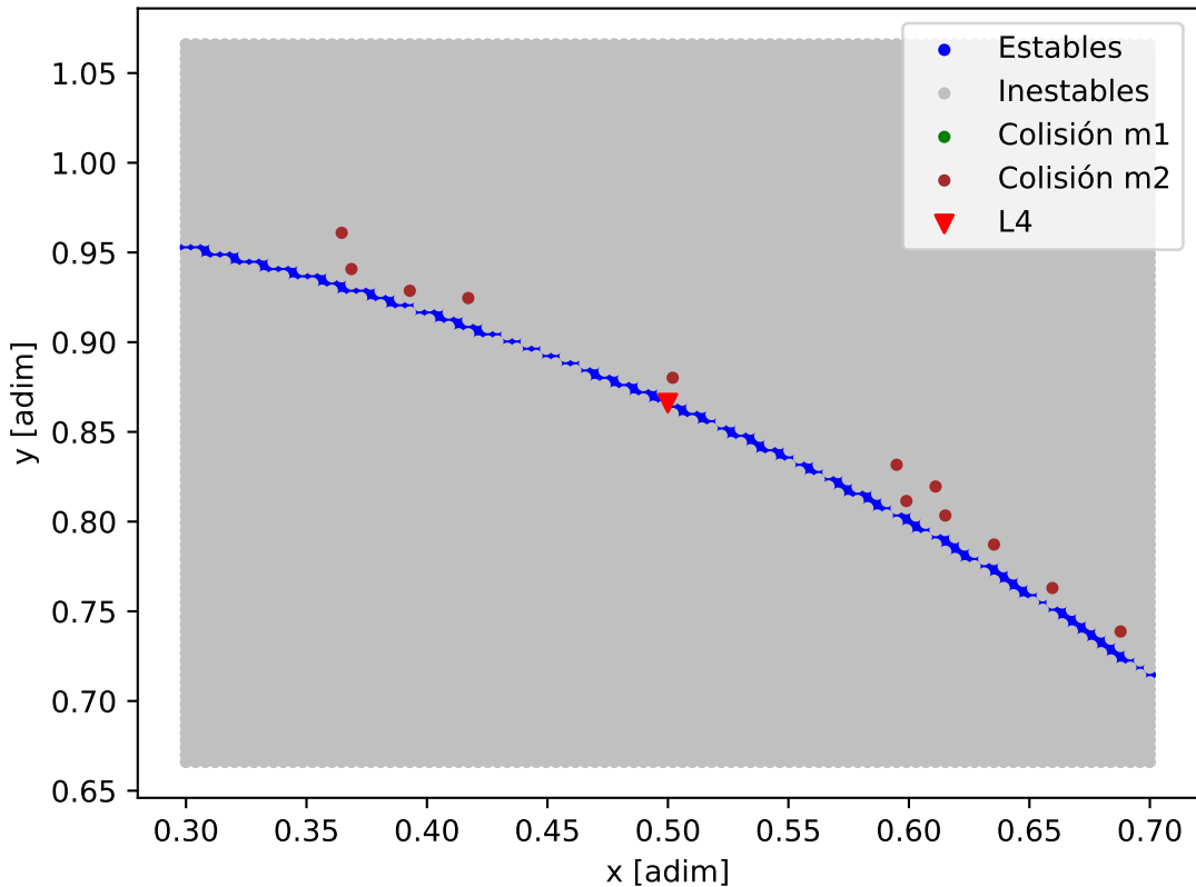
Mapa de estabilidad - HD_18143
