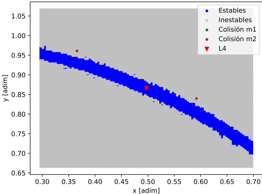
Mapa de estabilidad - HD_181433
