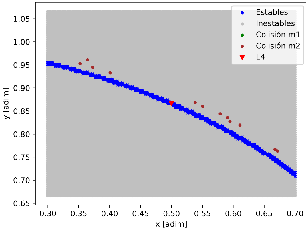
Mapa de estabilidad - HD_184010
