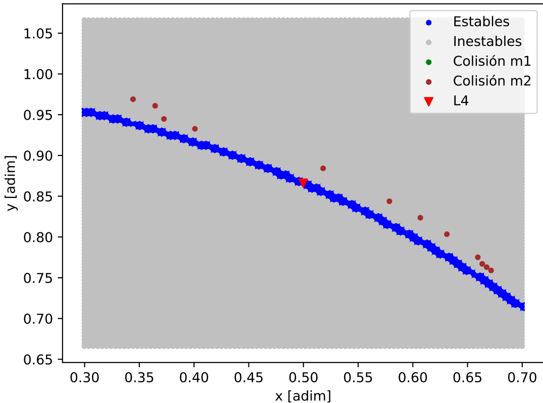
Mapa de estabilidad - HD_27894
