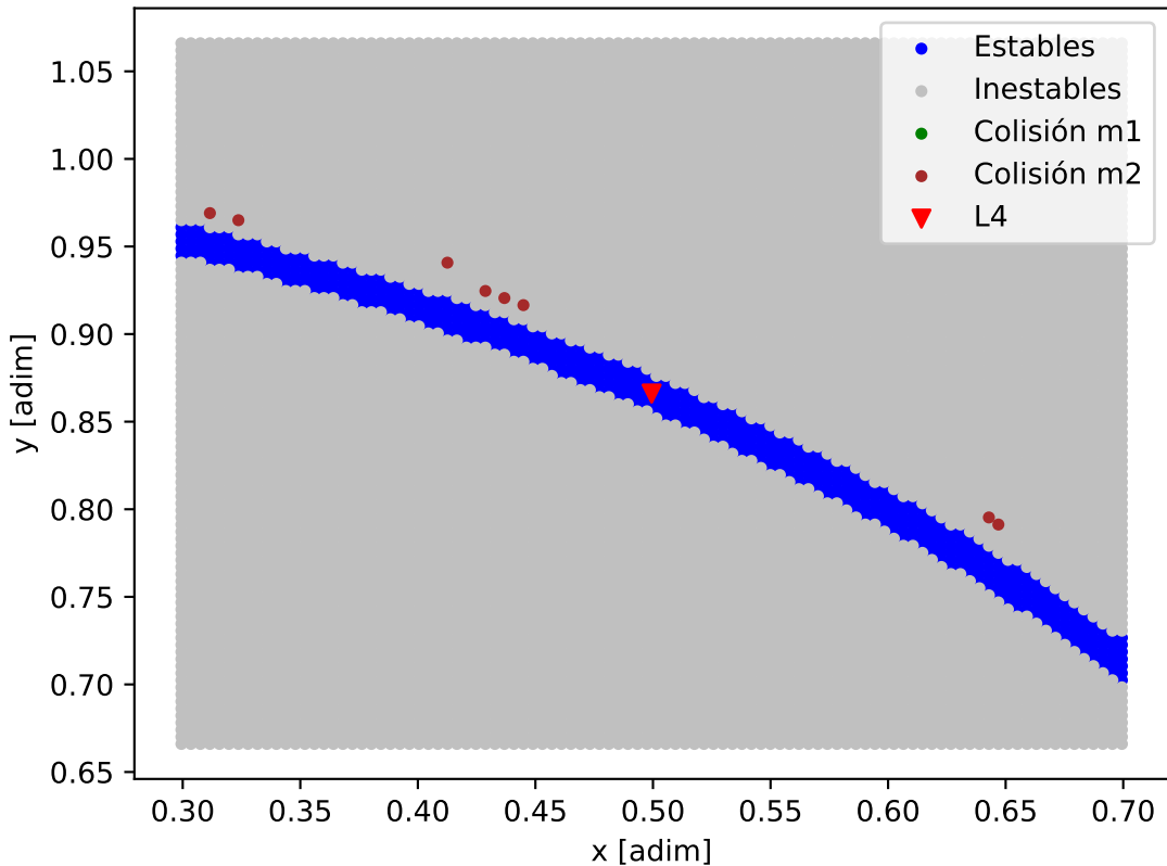
Mapa de estabilidad - HD_33142
