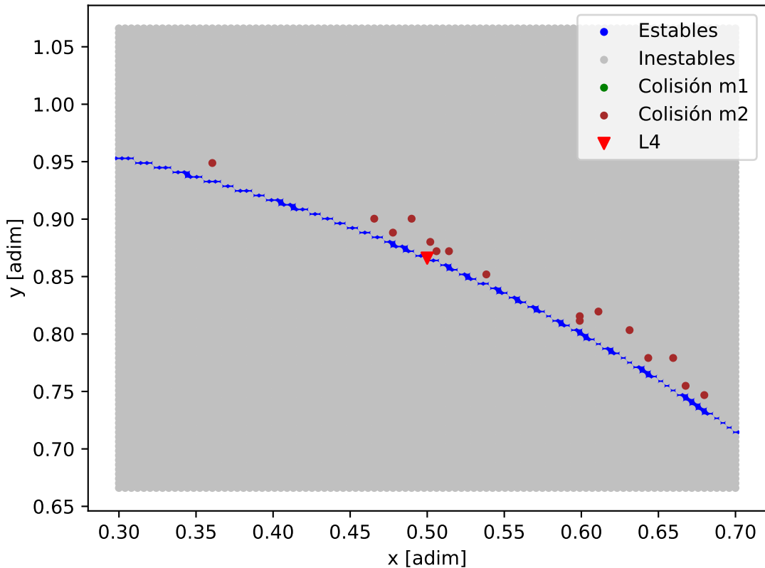
Mapa de estabilidad - HD_40307
