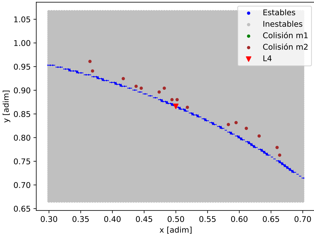
Mapa de estabilidad - HD_48948
