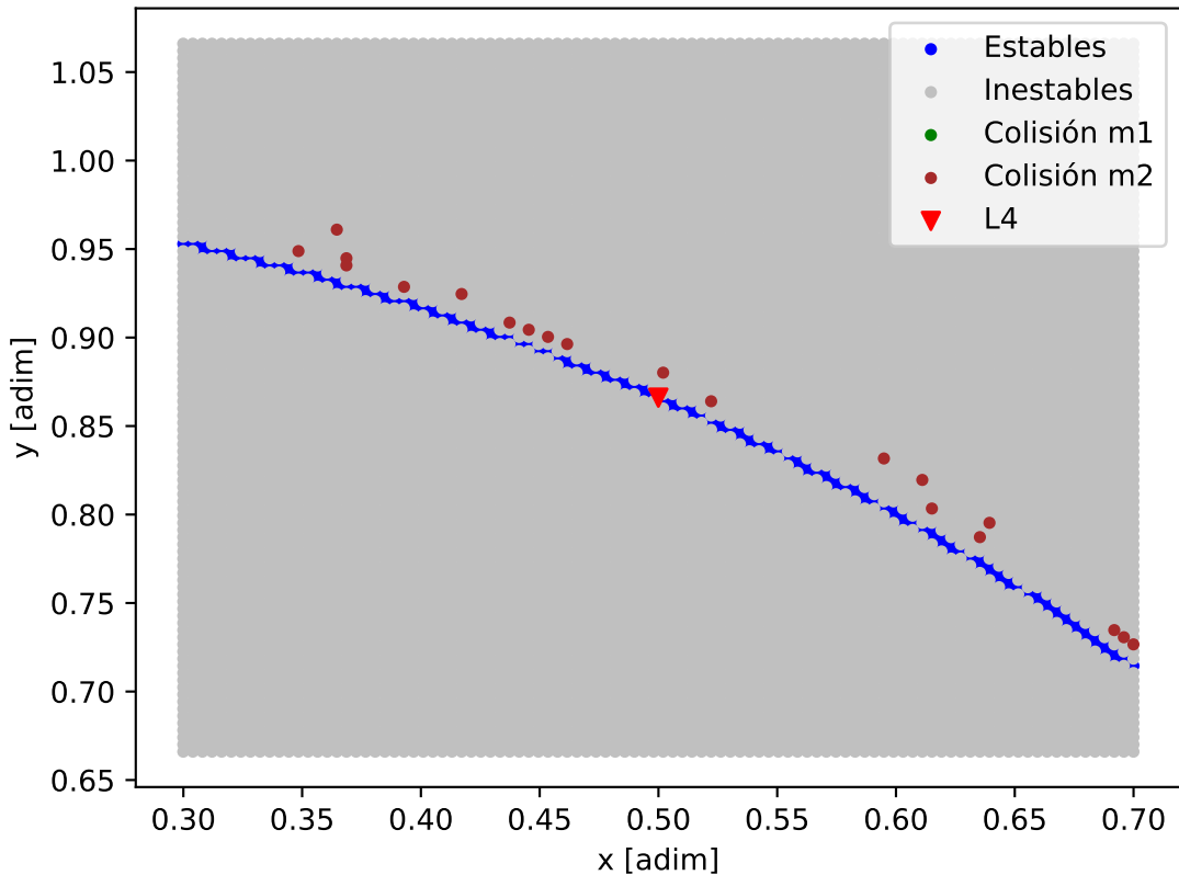
Mapa de estabilidad - HD_69830
