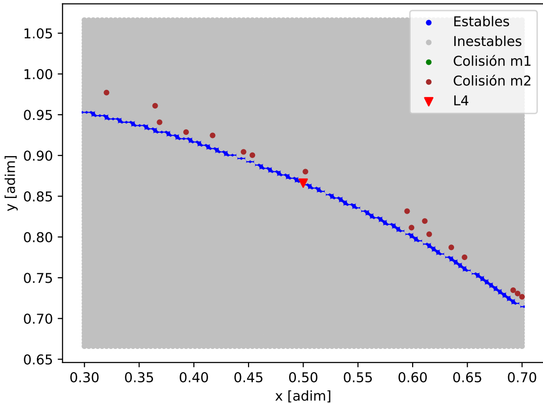
Mapa de estabilidad - HD_73583
